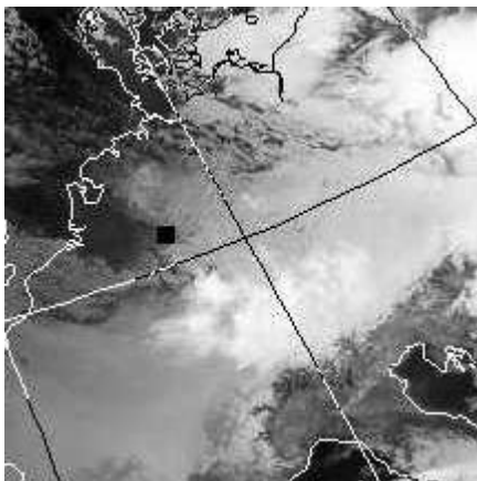
Abb. 1a, b: Satellitenbilder (Infrarot, Ausschnitte) von NOAA 14 vom 21.01.2000, 03.00 UT (oben) und 04.42 UT (unten). Das schwarze Quadrat markiert die ungefähre Lage von Bonn.
